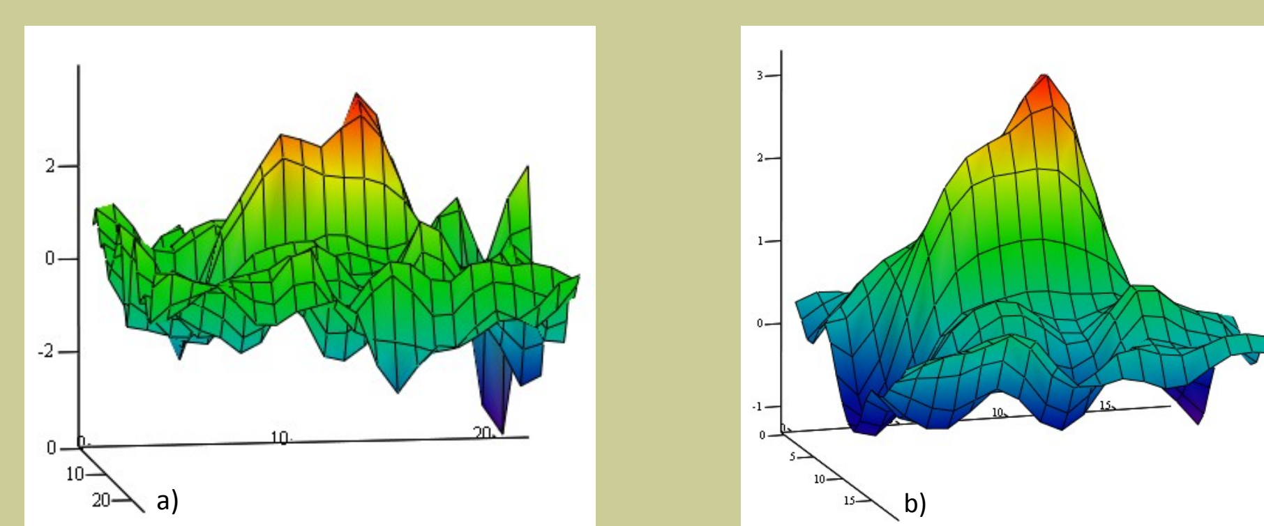
Lokaler Wärmestrom bei Blasenbildung durch Wärmeleitung vorher a) und nach Anwendung der Glättung nach GAUSS
