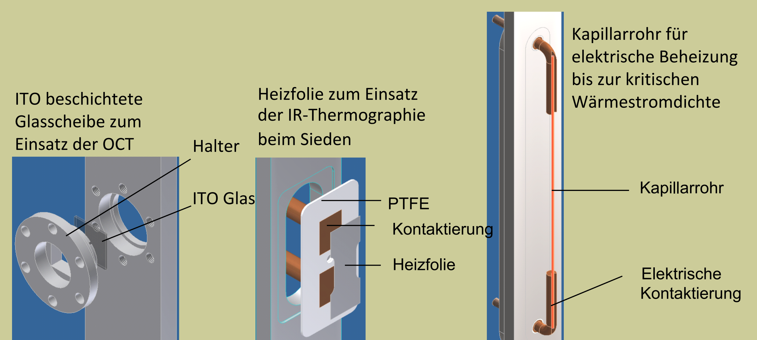
Aufbau der Versuchsanlage „unterkühltes Sieden“
