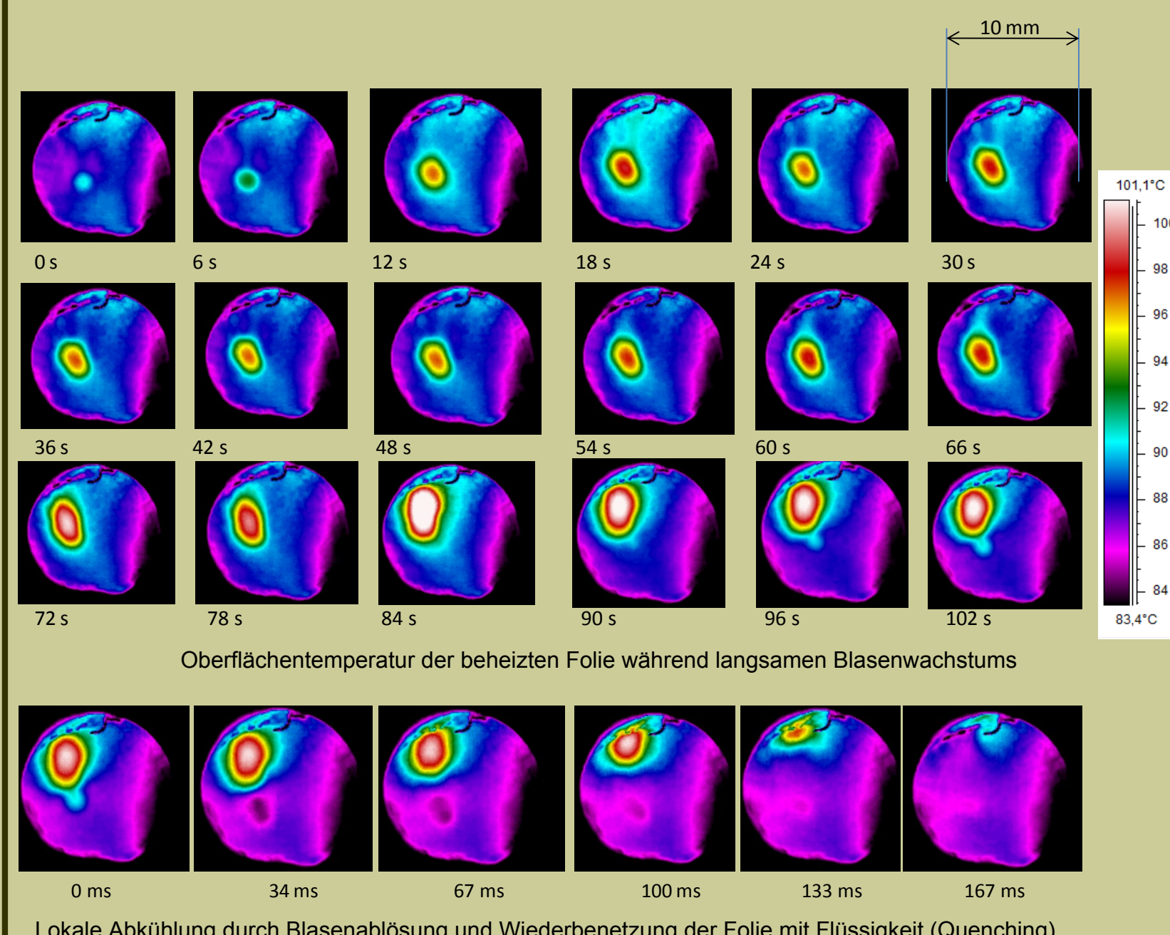
Lokale Abkühlung durch Blasenablösung und Wiederbenetzung der Folie mit Flüssigkeit (Quenching)
