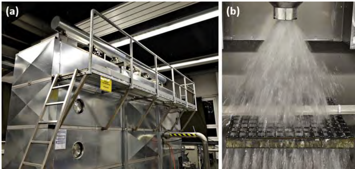
Abb. 4-54: Der Versuchsstand "Zittauer Strömungswanne" des IPM (a) dient u. a. der Analyse von Korrosionsprozessen an metallischen Komponenten, die von einem Leckstrahl beaufschlagt werden (b).
