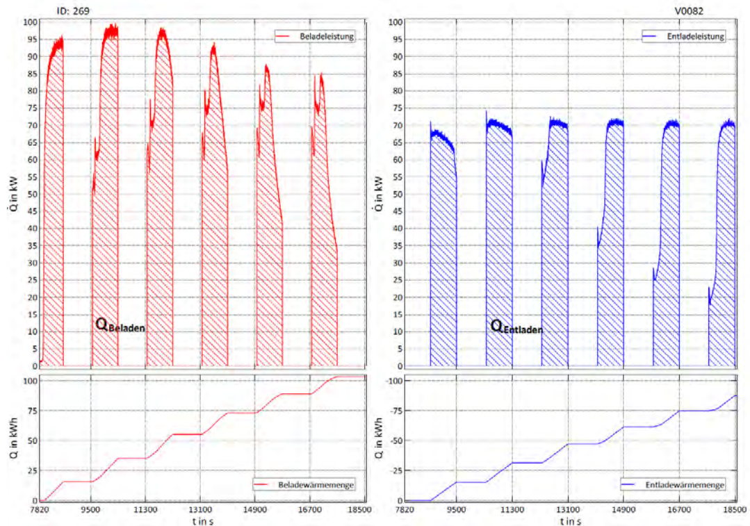
Abb. 4-2: Bilanzierung des GDVS bei mehrfacher Teilbe- und Entladung
