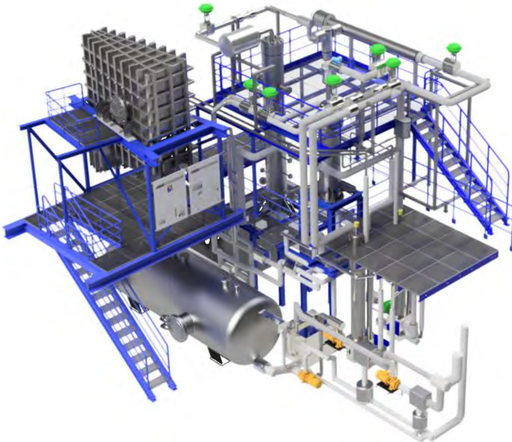
Abb. 4-53: Versuchsanlage THERESA des Zittauer Kraftwerklabors
