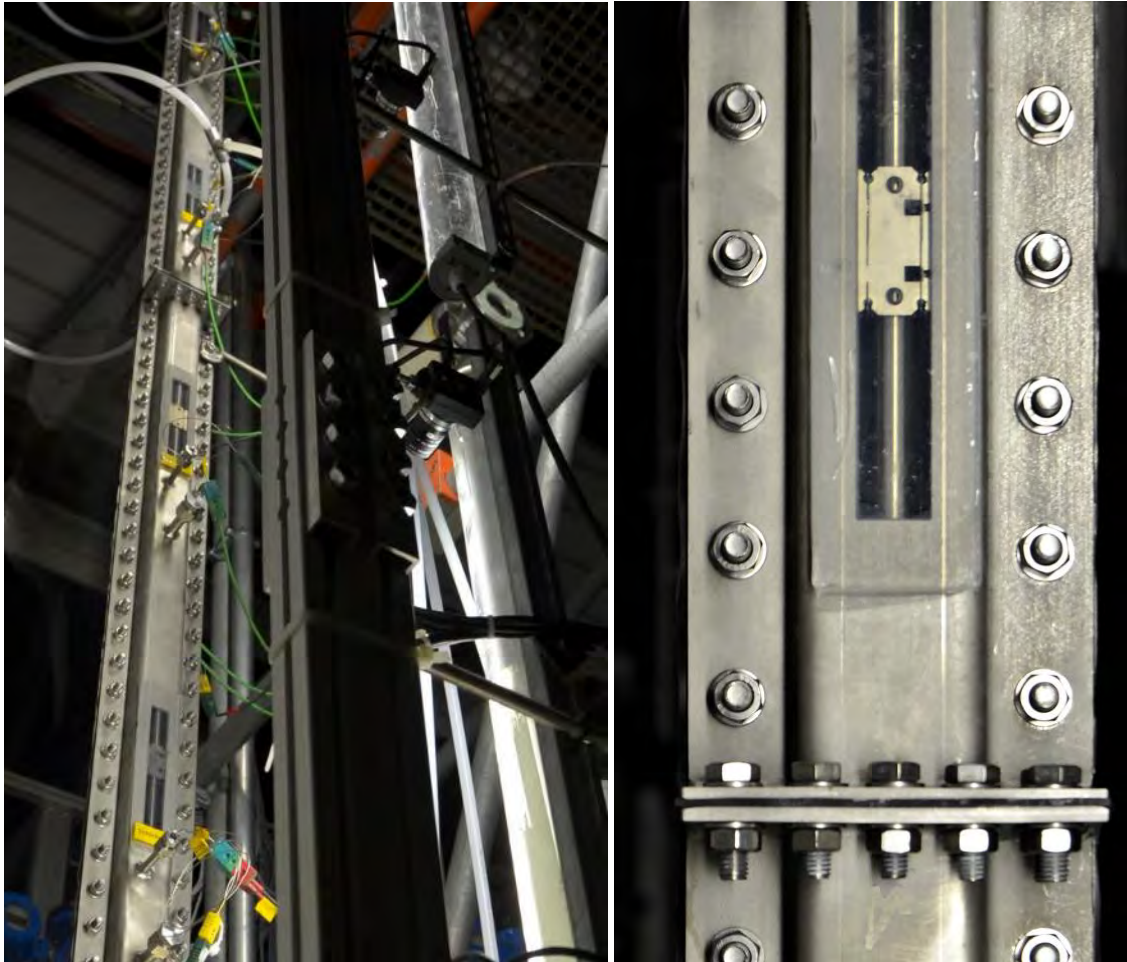
Abb. 4-12: Versuchsstandskomponente CORVUS (links); Edelstahl-Gehäuse mit 3x3-Heizstabkonfiguration in originaler Brennstablänge (rechts)
