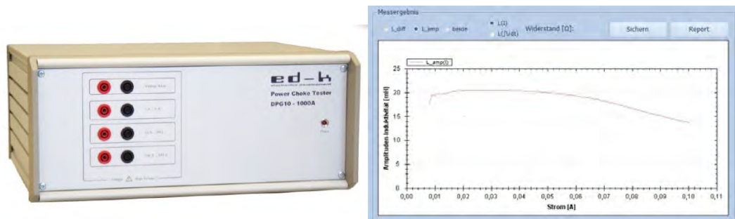
Abb. 4-25: Power Choke DPG 10 und Ergebnis einer Testmessung
