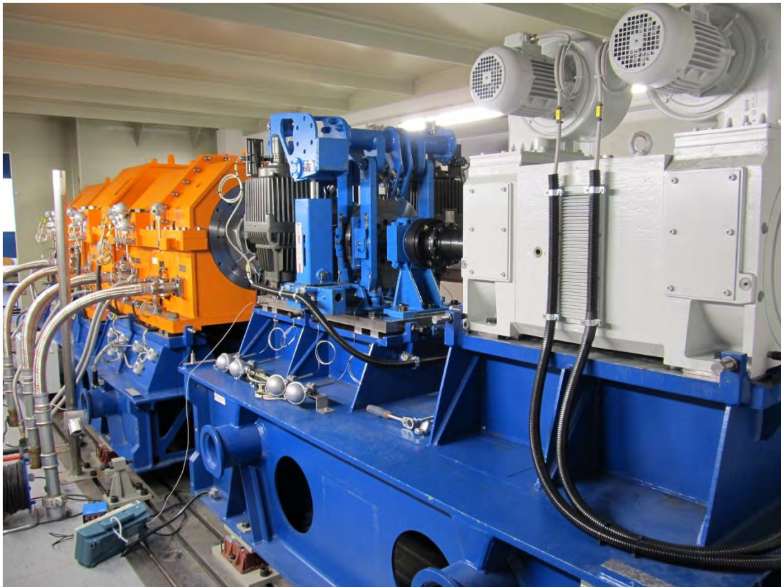
Abb. 4-22: Versuchsanlage Schmiermittelfreie Dampfturbine SFDT
