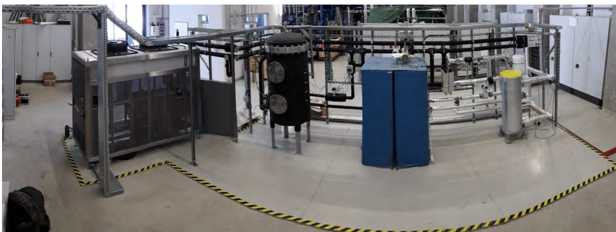
Abb. 4-28: Testfeld für Wärmespeicher
