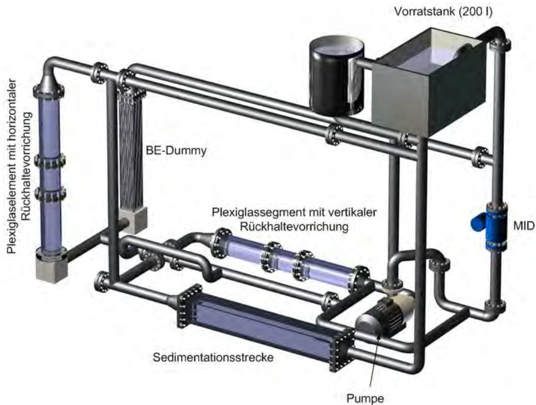
Abb. 4-8: Schematische Darstellung des Versuchsstands "Ringleitung II"
