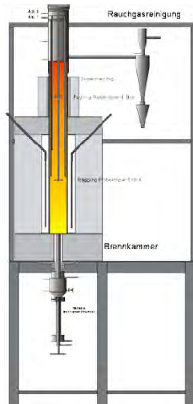
Abb. 4-31: Mikrobrennkammer MB 1500
