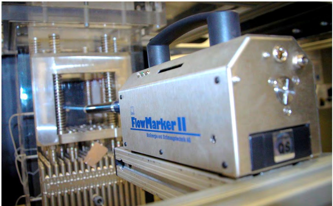
Abb. 4-10: Einsatz eines Strömungsmarkierers zur Visualisierung der vorherrschenden Strömungen
