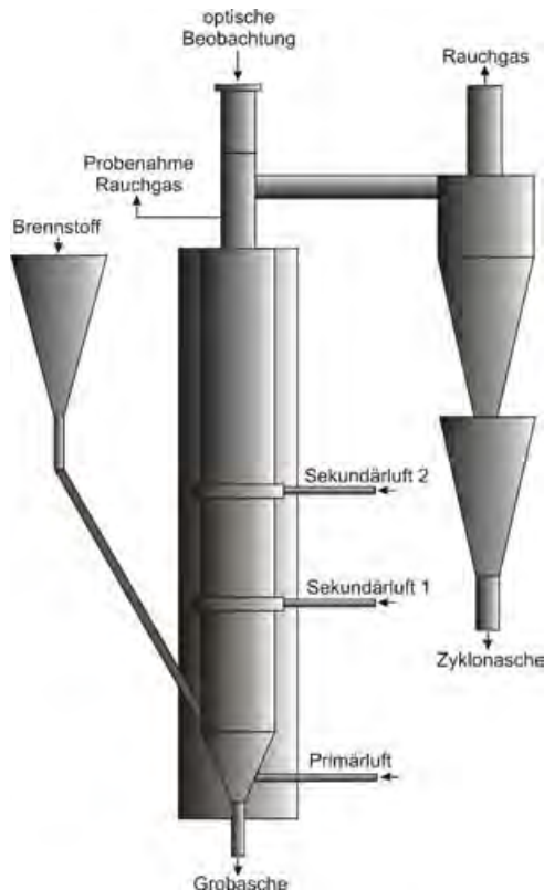
Abb. 4-32: Modell-Zyklonfeuerung ZBK 2
