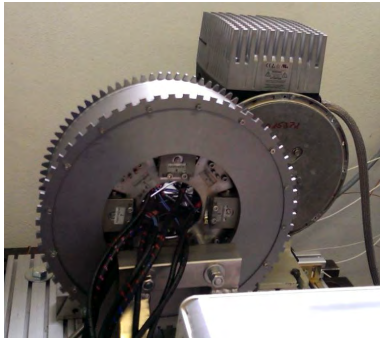
Abb. 4-23: Versuchsstand Momentenlager ZML320
