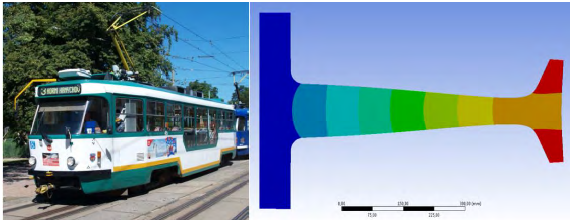
Abb. 4-18: Straßenbahn T3 und Analyse der Verformungen am Schwungrad (Lavalscheibe)
