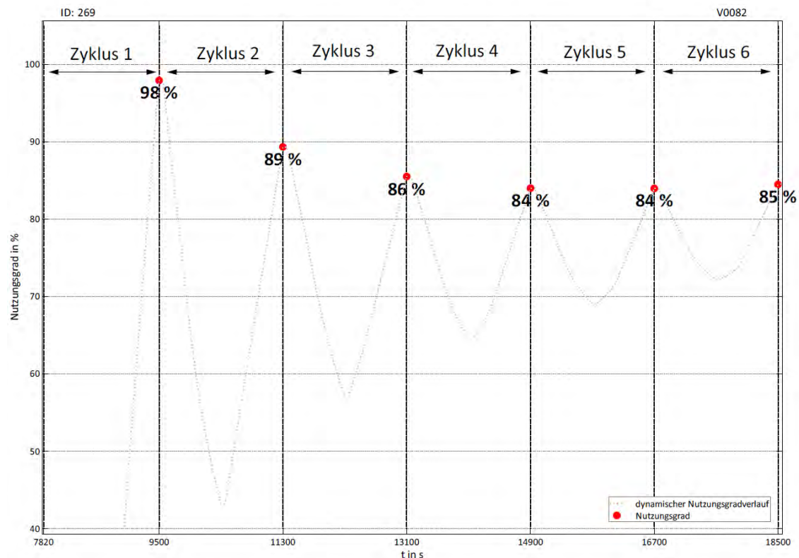
Abb. 4-3: dynamischer Nutzungsgradverlauf des GDVS bei mehrfacher Teilbe- und Entladung
