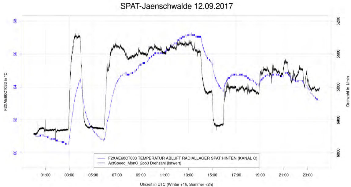
Abb. 4-17: Lastabhängiger Temperaturverlauf am hinteren Radiallager
