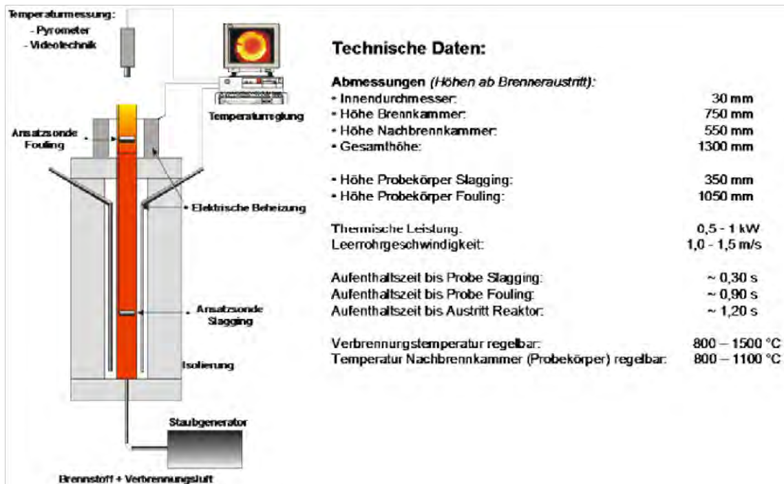
Abb. 4-30: Mikroverbrennungsreaktor MR 1500
