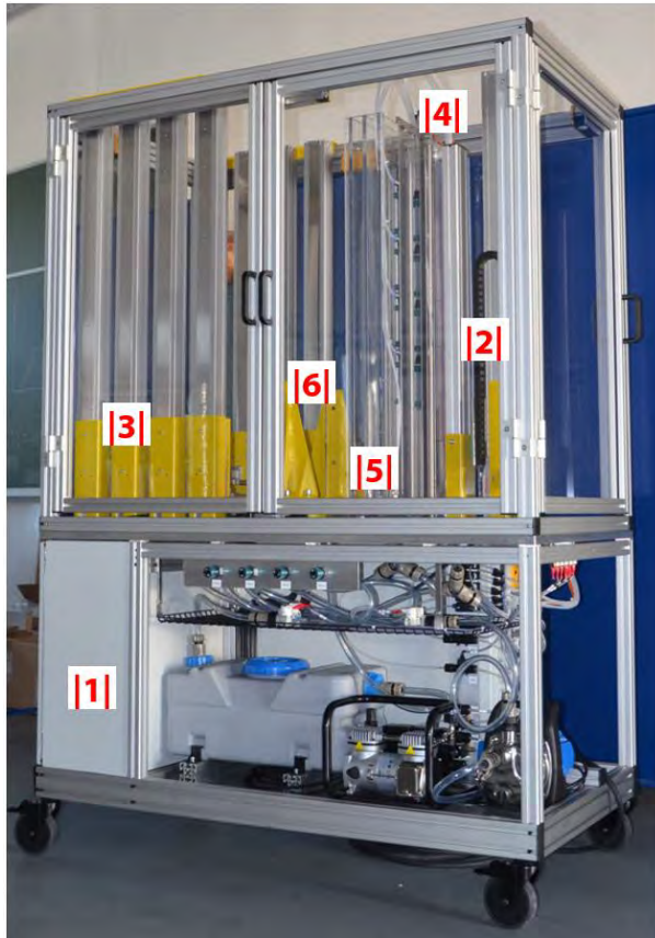
Abb. 4-5: Versuchsstand Nicole
